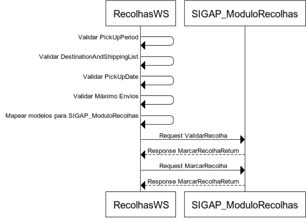
Figura 2 - CompletePickUp - Marcação de Recolha
