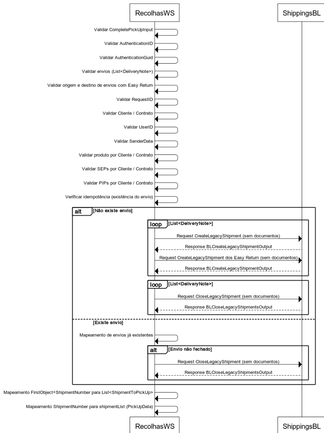
Figura 1 - CompletePickUp - Criação e fecho de envios
